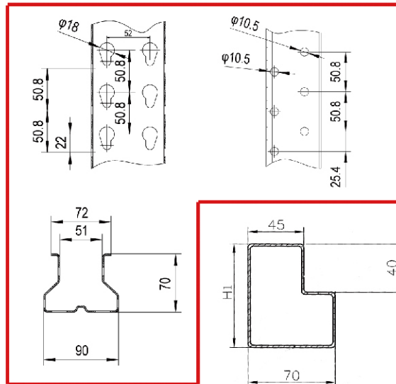
Upright Frame
